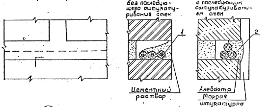
Рис.1 Закрите прокладання кабелів по негорючих основах (в бороздах, під мокрою штукатуркою)
